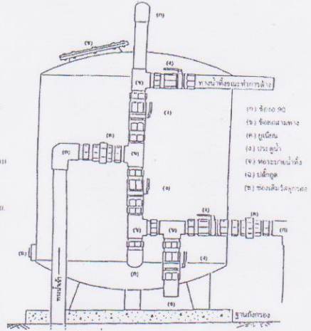
รูป อุปกรณ์ภายนอกของถังกรอง (กรมทรัพยากรน้ำบาดาล, 2551)
